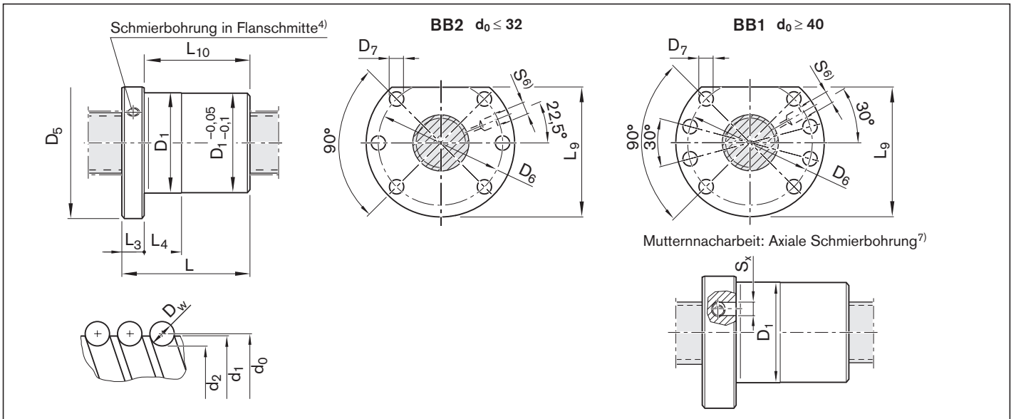
7) Die axiale Schmierbohrung S_x liegt immer auf dem Teilkreis D_6 der Muttereinheit.
